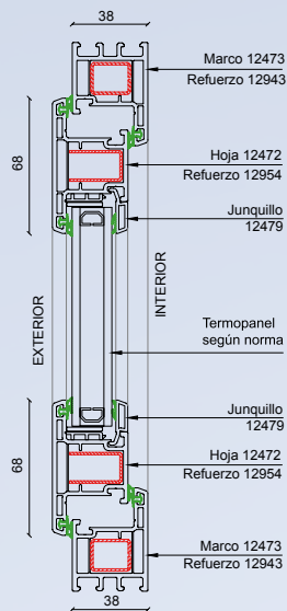
Detalle 1
